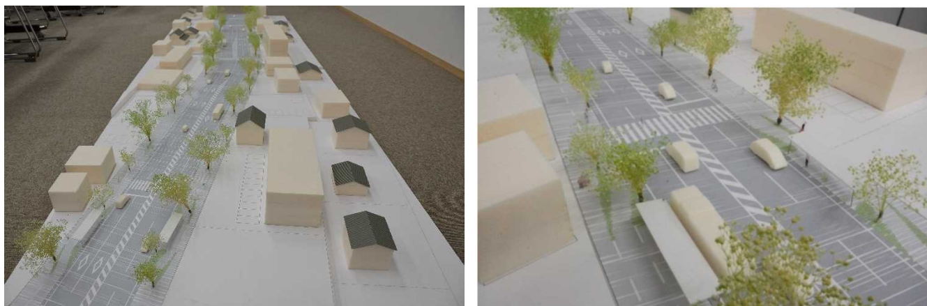
ましきラボが製作した 27m 県道の道路模型例
