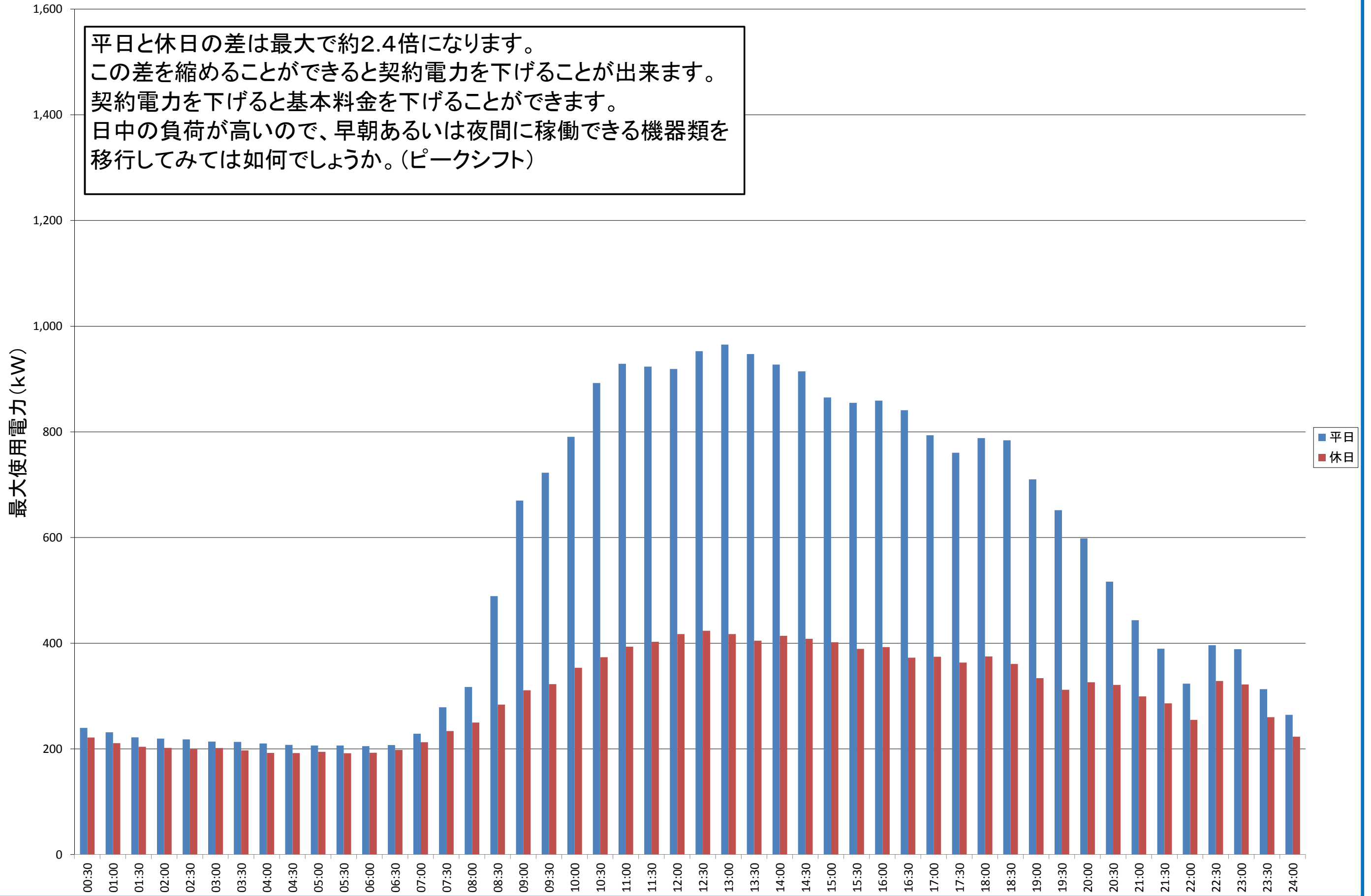
黒髪北キャンパス 1月の時間帯別最大使用電力平均値
