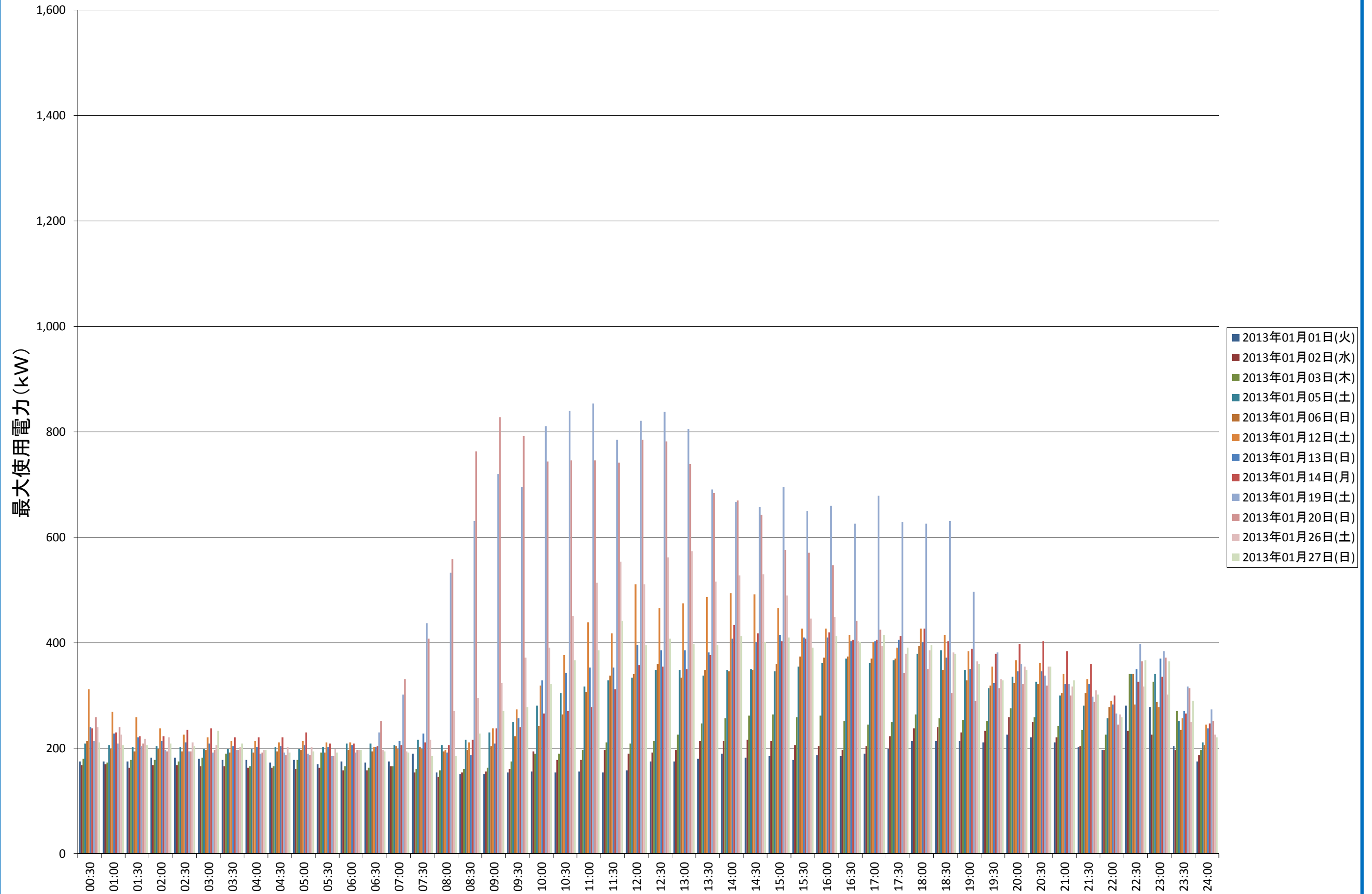
黒髪北キャンパス 1月の時間帯別最大使用電力(土日祝)
