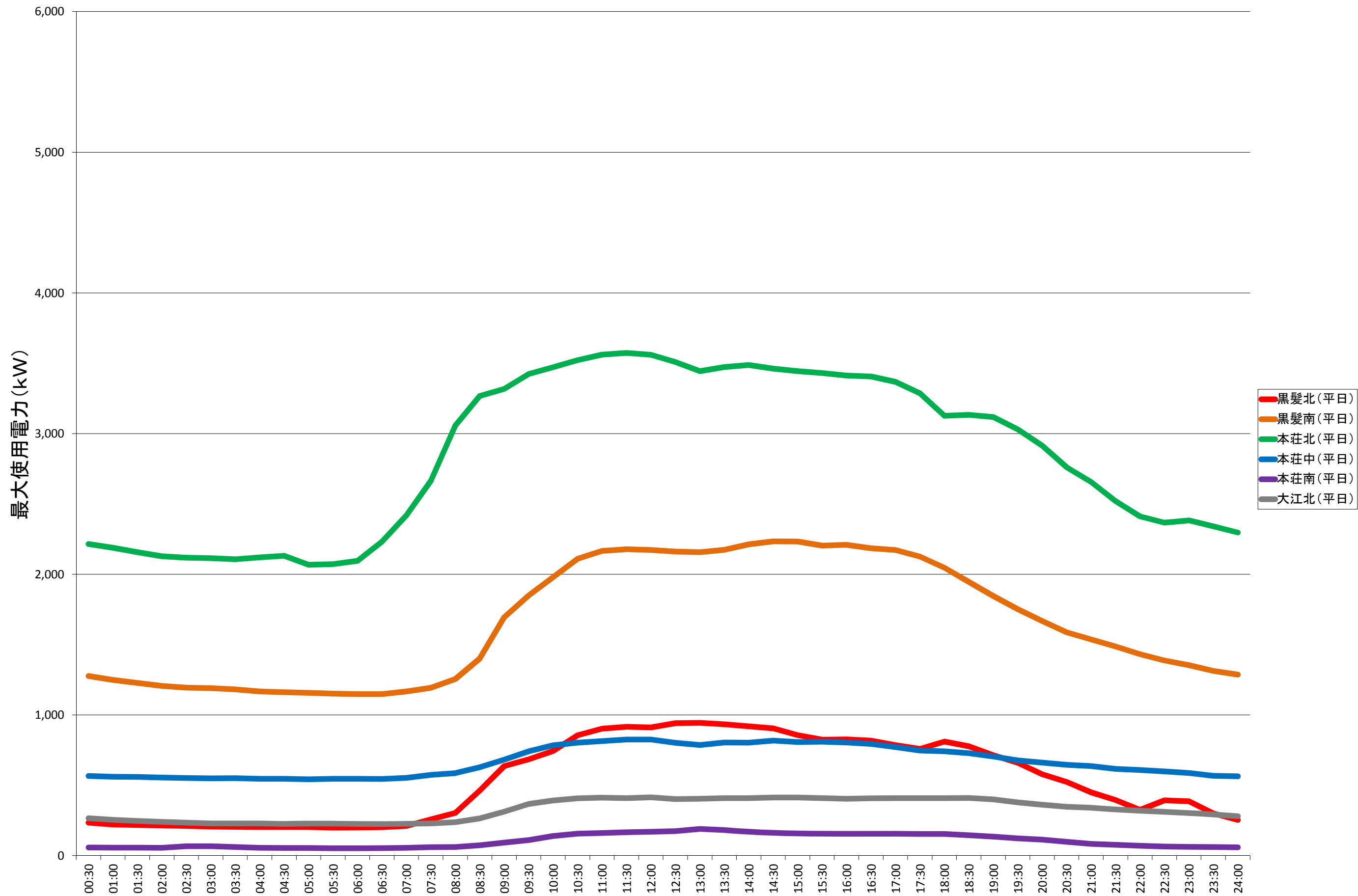
主要6キャンパス 12月の時間帯別最大使用電力平均値
