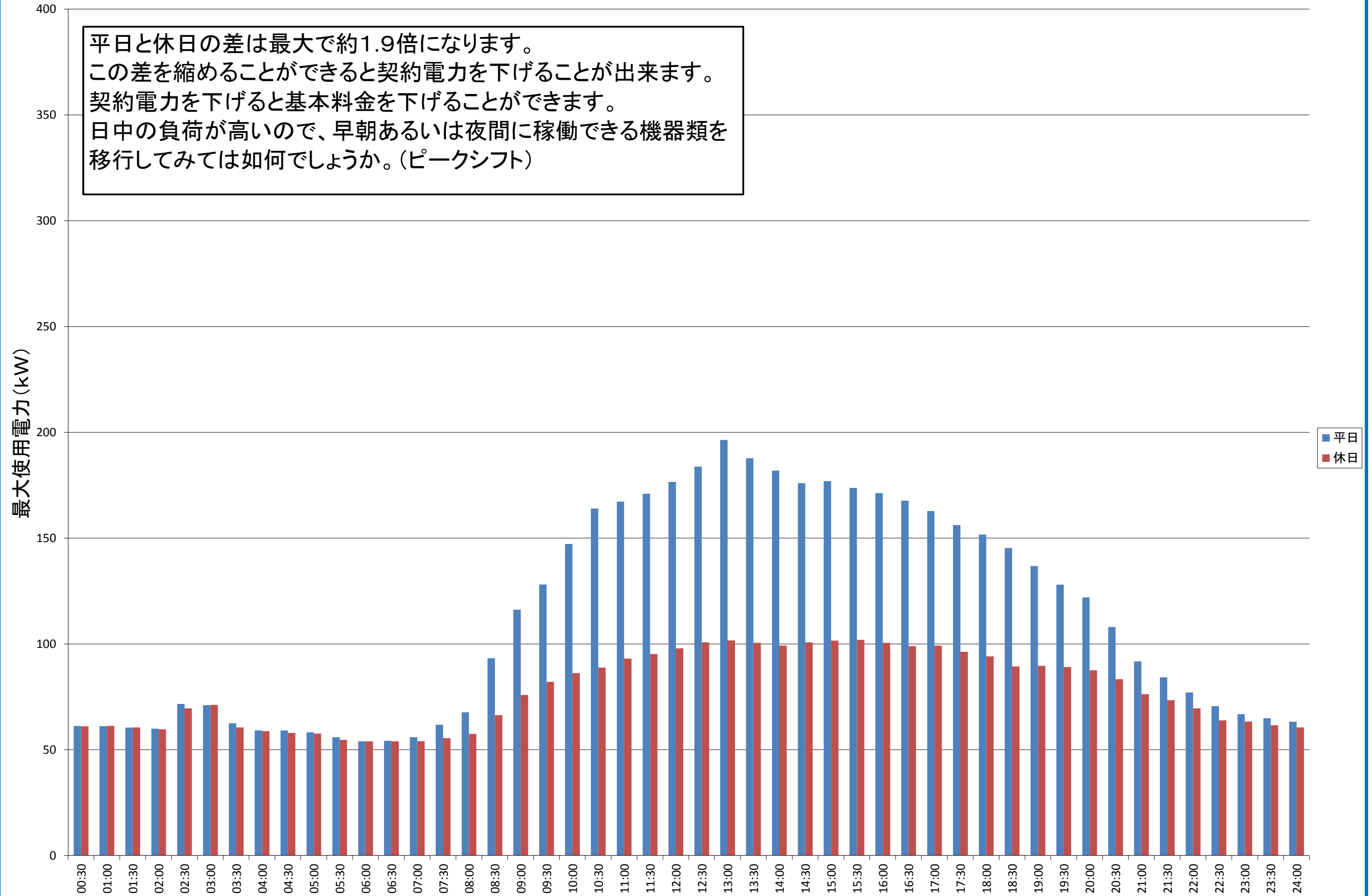
本荘南キャンパス 7月の時間帯別最大使用電力平均値
